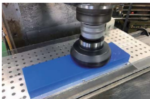
吸着治具でワークを固定、板厚仕上げ加工
