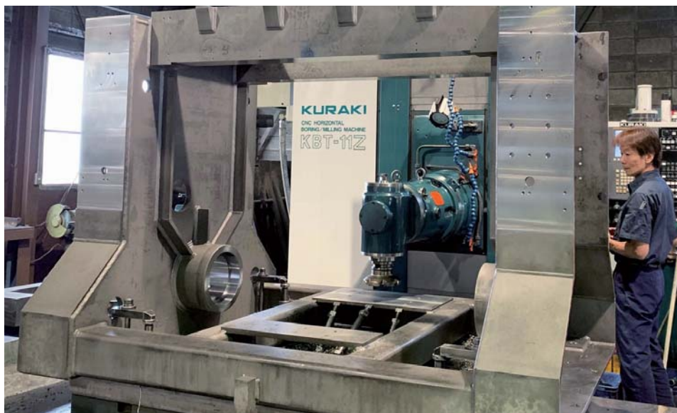
アタッチメントを使った切削作業
