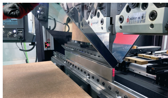
鋼板を曲げて立体成形を行う
