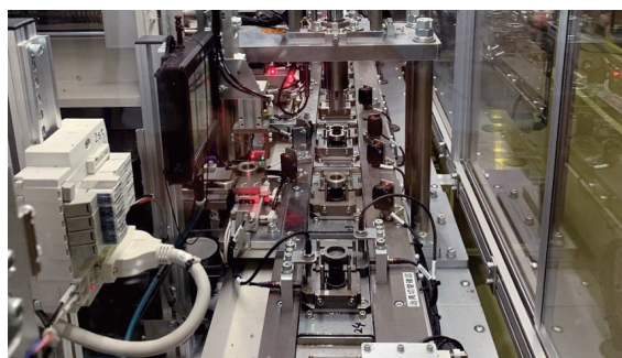
プレスベアリング自動組立機
