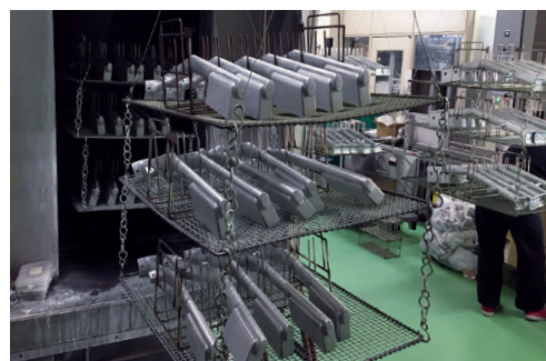
化成被膜による防錆処理、密着の向上処理
