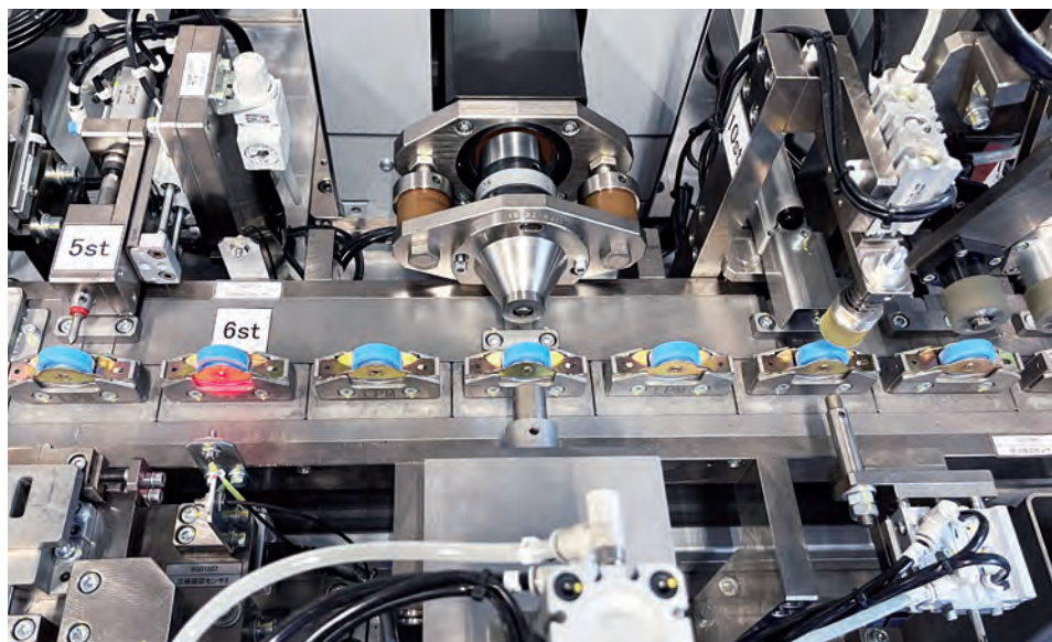
共同開発したハイスピード自動組立機
