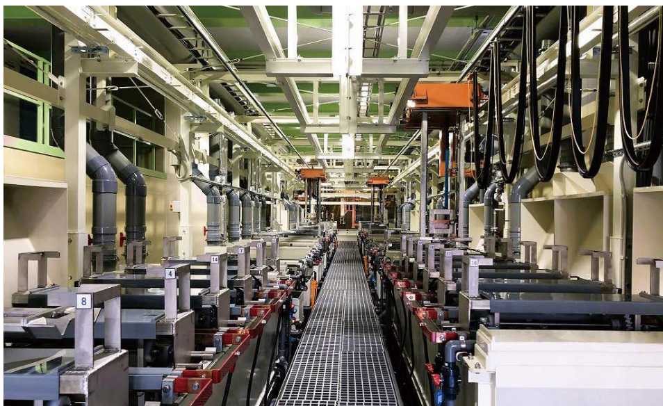
巽中工場(大阪市生野区)の自動めっき加工ライン
