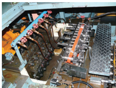
横型多段式鍛造機械ナットフォーマー「NF-530」
