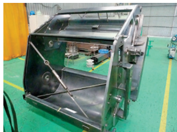
1mm単位の精度でつくられた塵芥車部品
