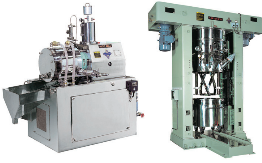
微分散機「ピコミル」(左)、混合混練機「プラネタリーデスパ」(右)
