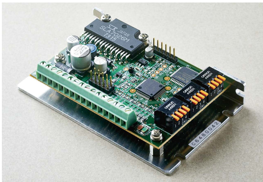
2相モータドライバ製品の一部
